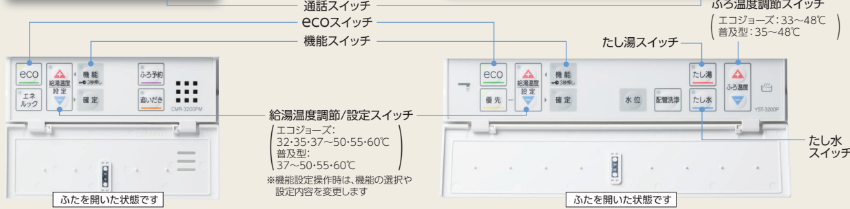
外形寸法 高120×幅128×奥20(mm) 非防水形
