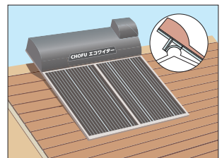
④ 簡易棟こし設置
