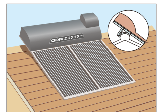
④ 簡易棟こし設置 ※2
