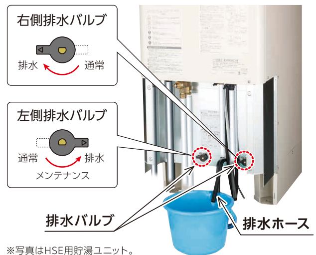
※写真はHSE用貯湯ユニット。
