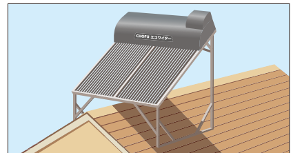
※1 ③棟またぎ設置(東西向屋根用架台)
