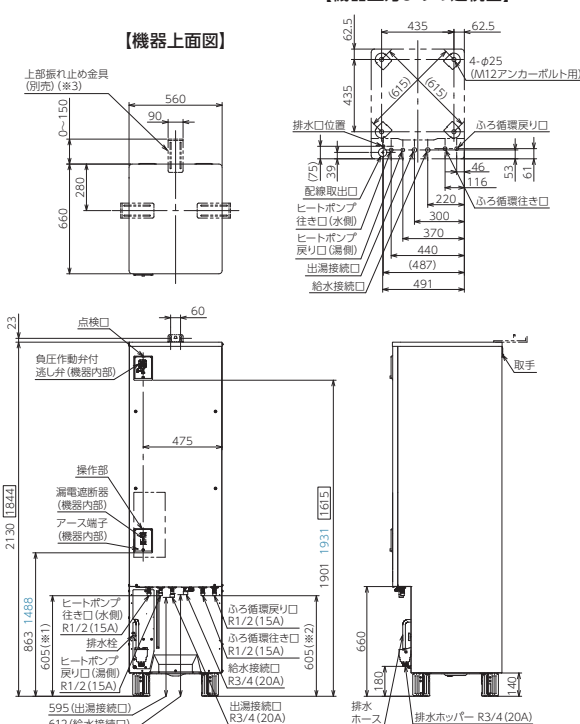
【機器上方よりの透視図】
