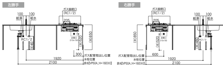
●側面図
