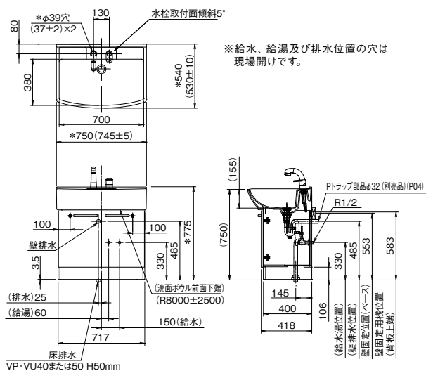
SK-753NSS
