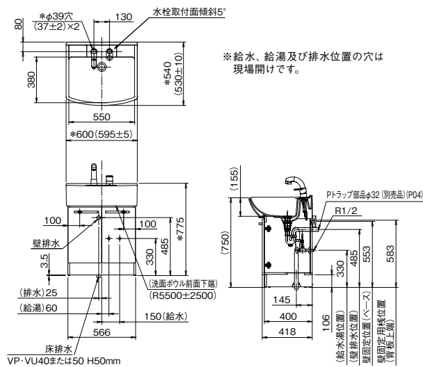
SK-603NSS
