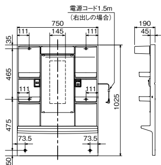
MK-750NL
