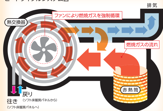
ヒートサイクルシステム図
