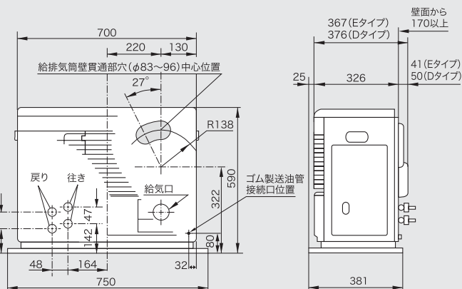
UFH-6432UKF
