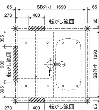
排水管(CR/SR)低脚仕様
