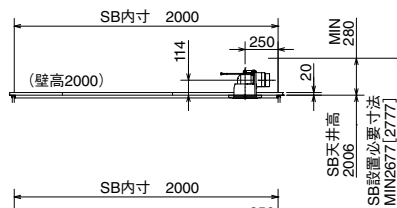
■標準仕様・高脚仕様立面図
