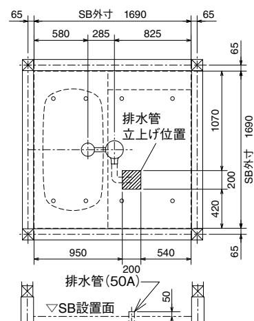
排水管(CL/SL)低脚仕様
