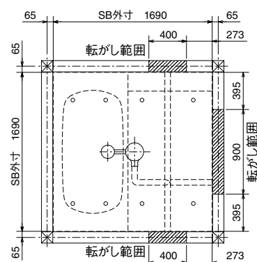
排水管(CL/SL)低脚仕様
